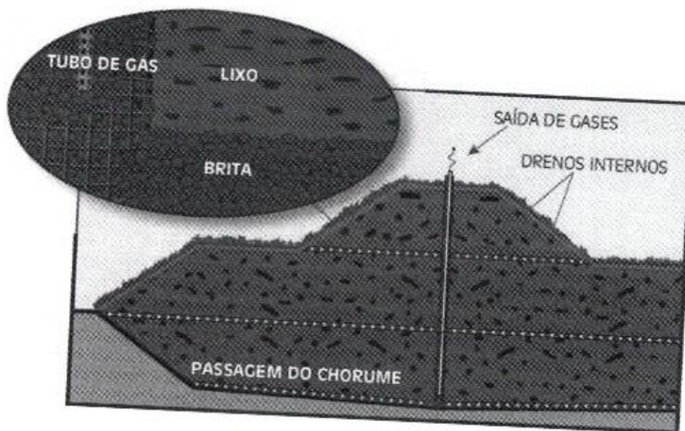
Figura 03- Ilustração da célula finalizada.
