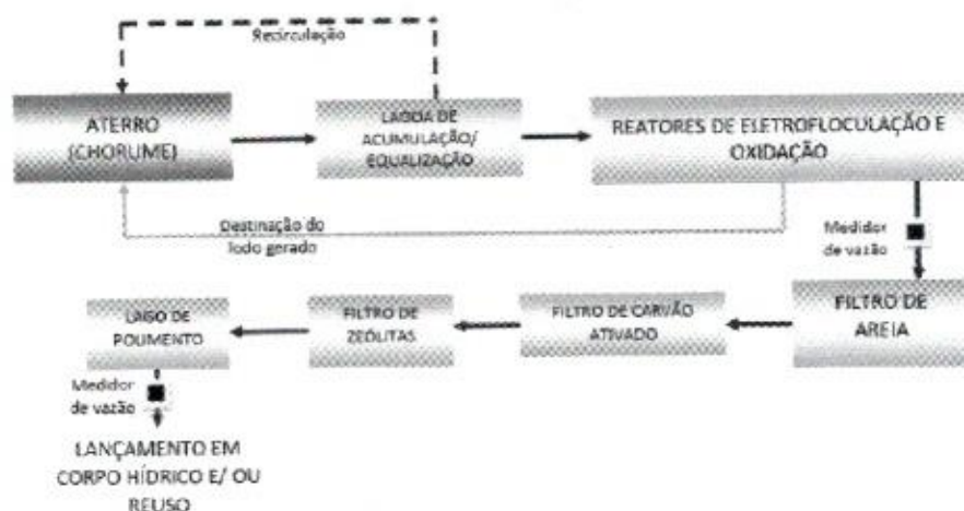
Figura 3.35: Fluxograma da ETE do empreendimento.
