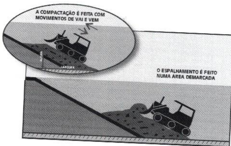
Figura 02- Ilustração da compactação dos resíduos na célula.
