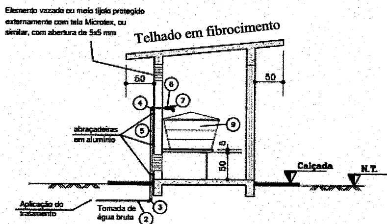
Casa de química Tipo E: Corte C - Entrada de água bruta Escala: 1:50
