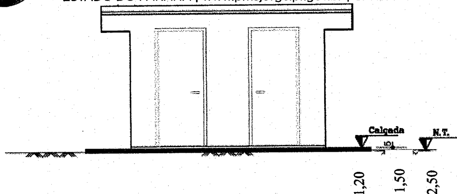
Casa de química Tipo E: Fachada principal Escala: 1:50
