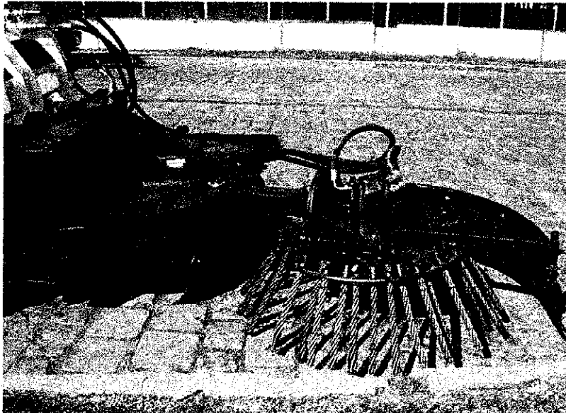
O acessório é facilmente instalado através do sistema de engates rápidos da carregadeira.
